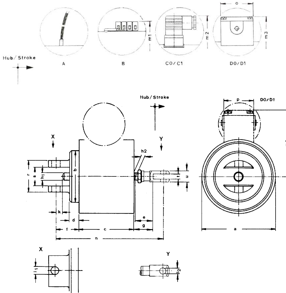
Abmessungs-Tabelle / Dimension Table [mm]
